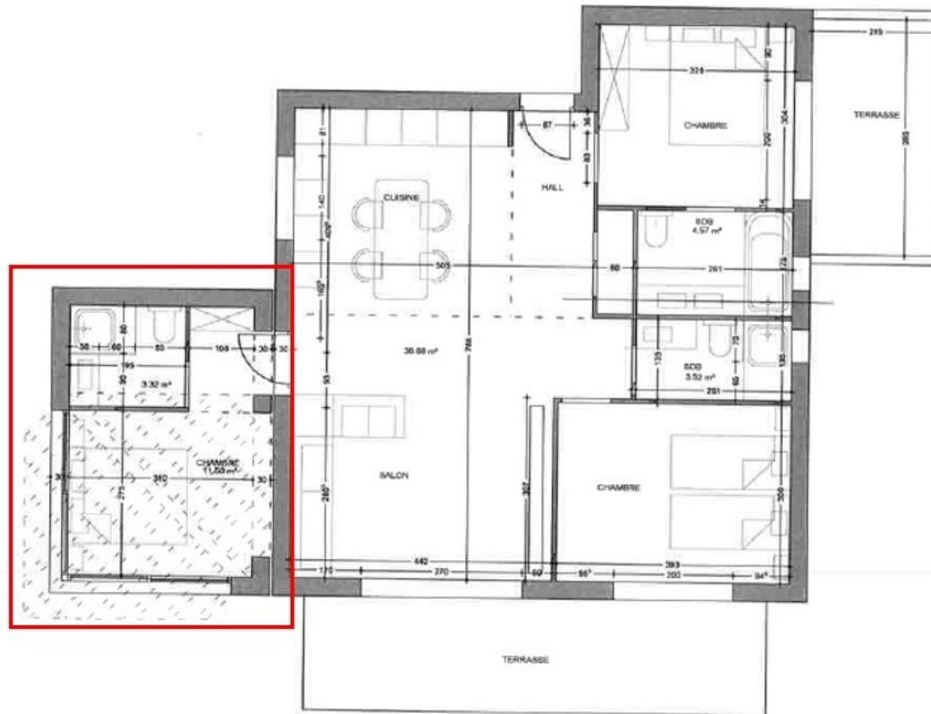
PROJET 1/100°
